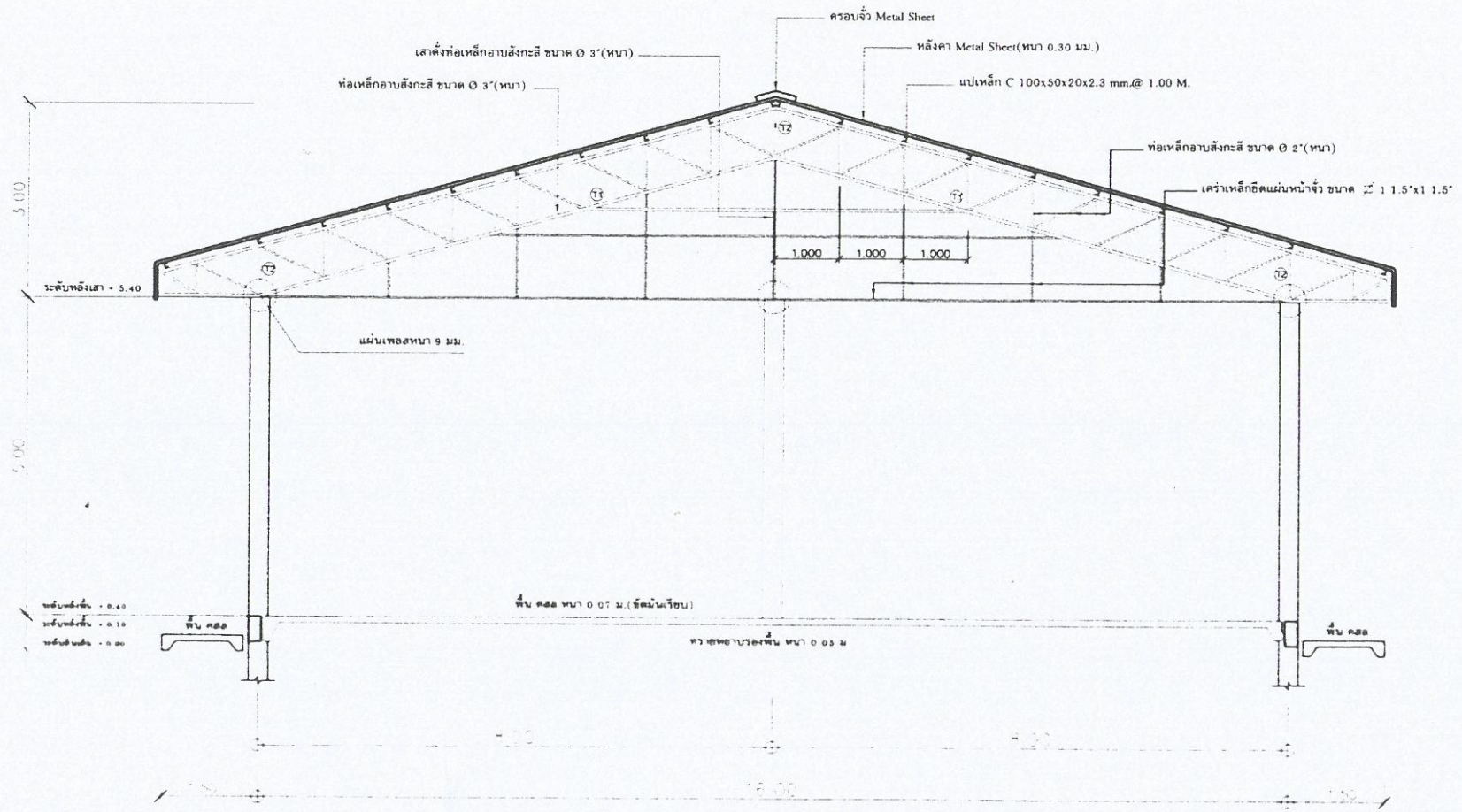
รูปตัด A - A มาตรฐาน 1 :
